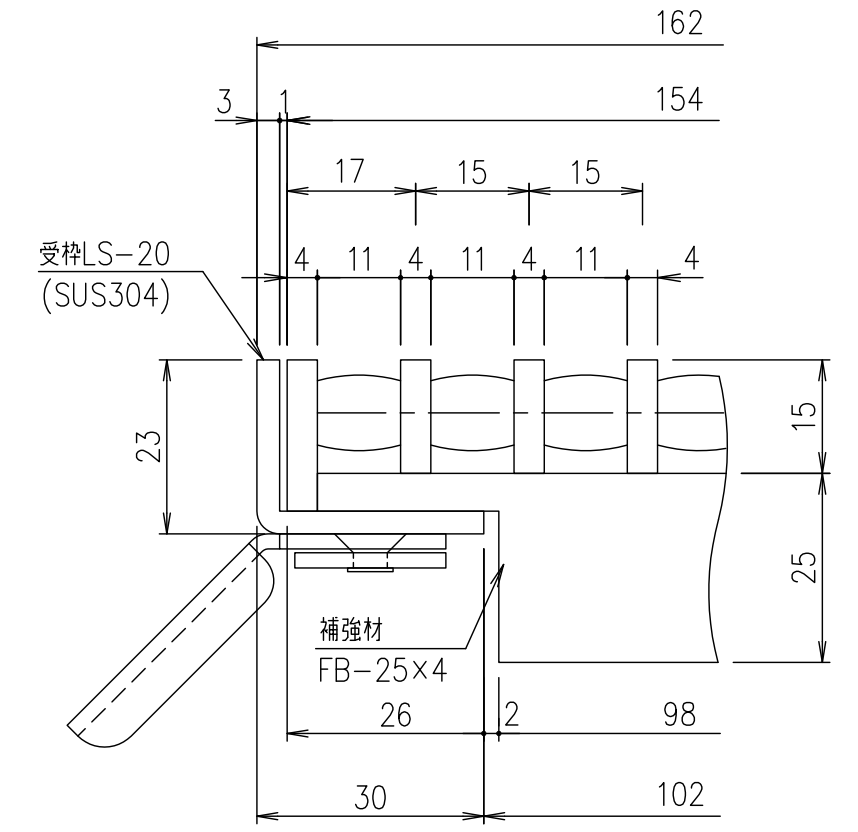
受枠断面・メインバーピッチ詳細図 S=1/1
