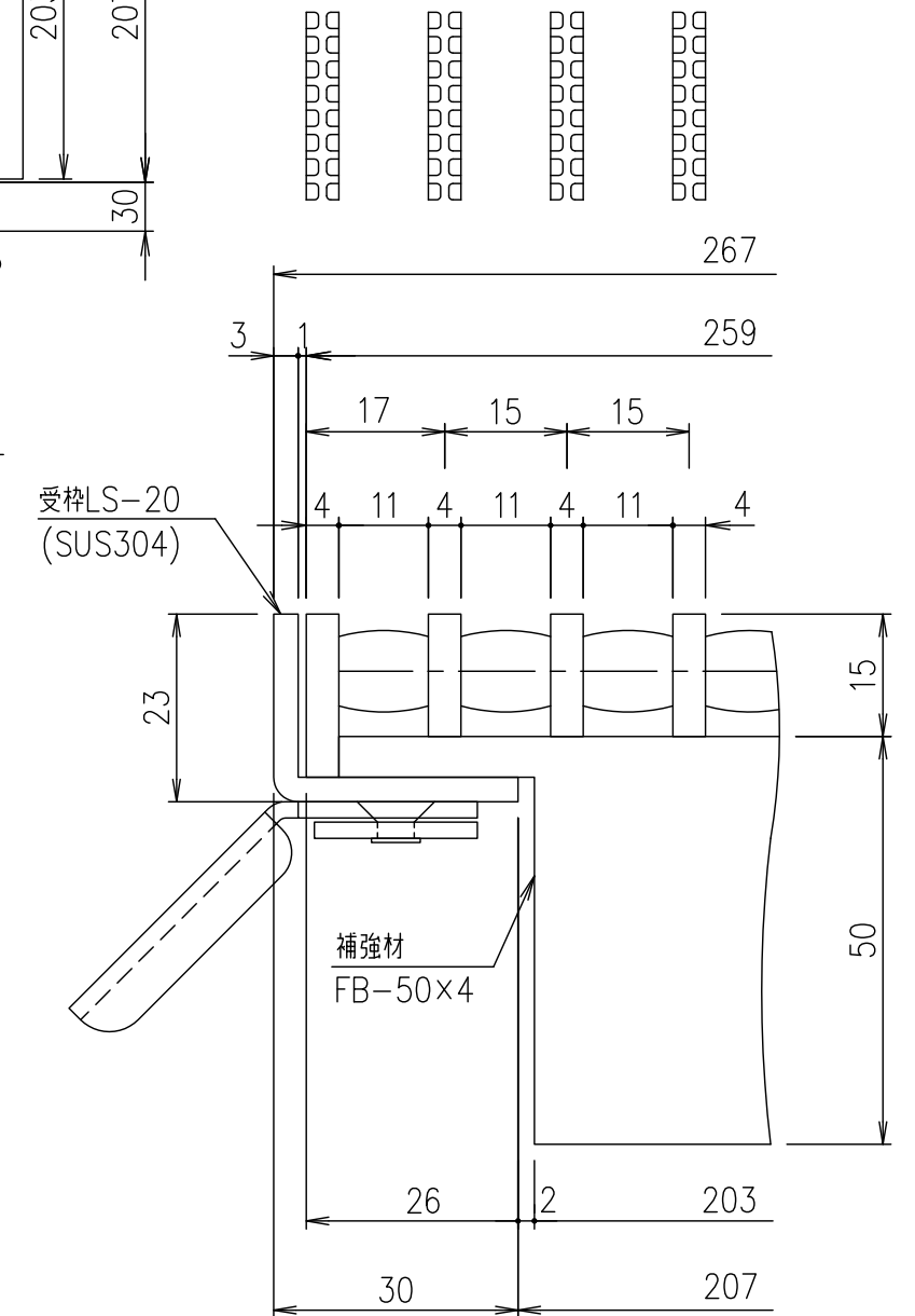
受枠断面・メインバーピッチ詳細図 S=1/1
