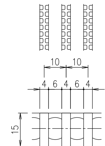
メンバーピッチ詳細図 S=1/1
