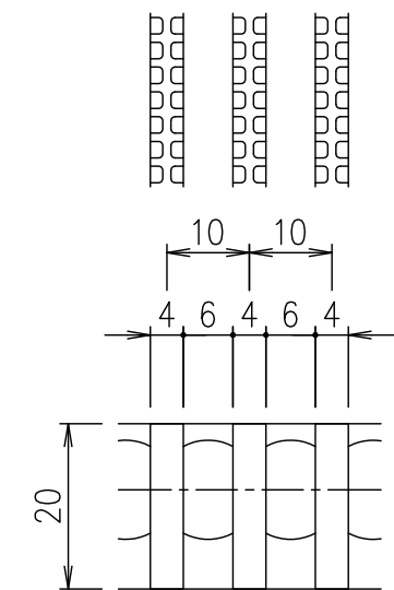
メンバーピッチ詳細図 S=1/1
