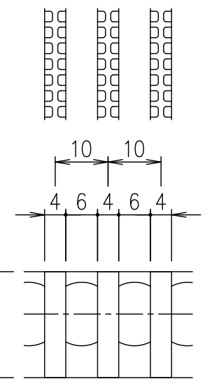
メインバーピッチ詳細図 S=1/1
