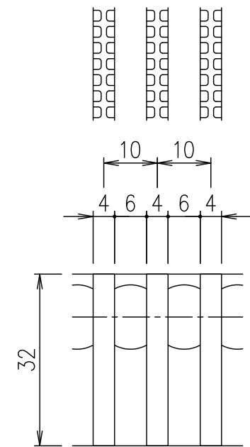
メンバーピッチ詳細図 S=1/1
