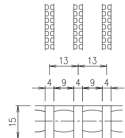
メンバーピッチ詳細図 S=1/1
