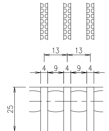
メンバーピッチ詳細図 S=1/1
