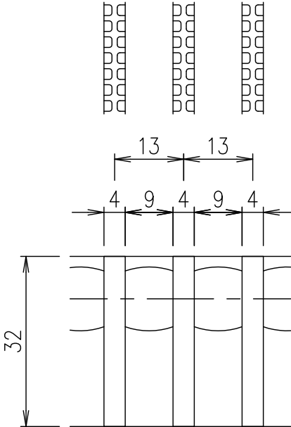
メインバーピッチ詳細図 S=1/1
