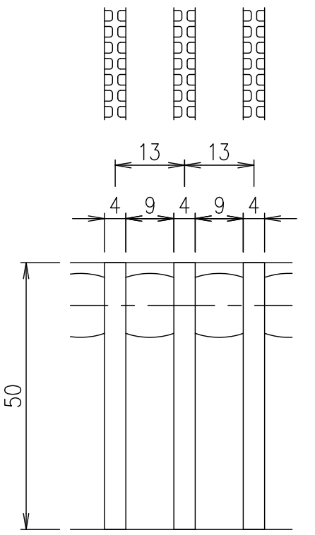
メインバーピッチ詳細図 S=1/1
