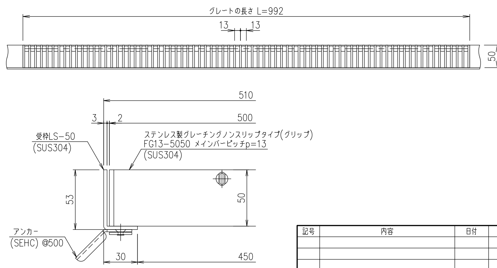
受枠断面詳細図 S=1/2
