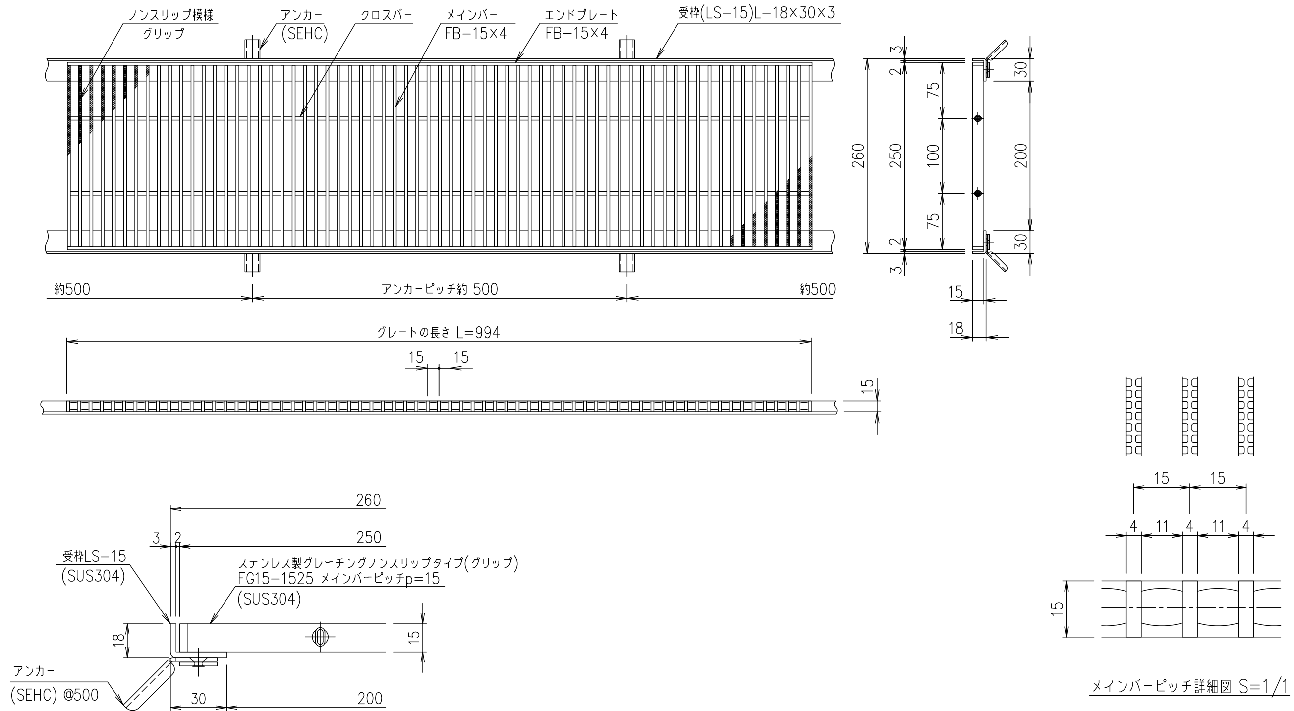
受枠断面詳細図 S=1/2
