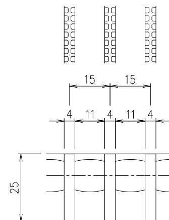
メンバーピッチ詳細図 S=1/1
