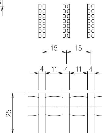
メンバーピッチ詳細図 S=1/1
