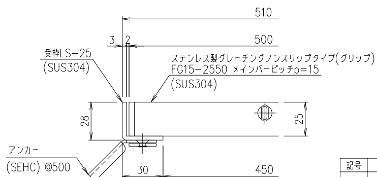
受枠断面詳細図 S=1/2
