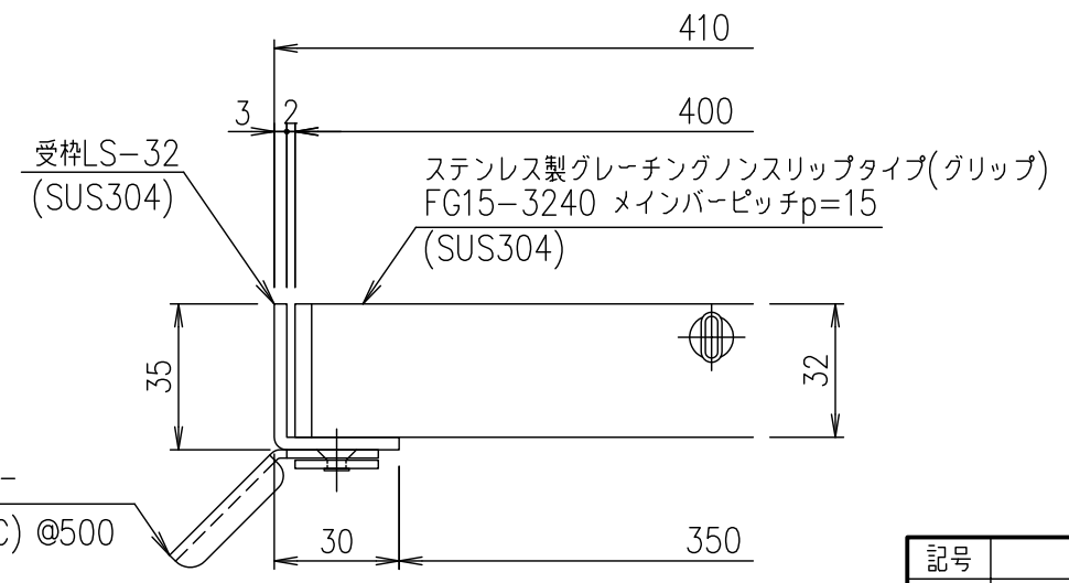
受枠断面詳細図 S=1/2
