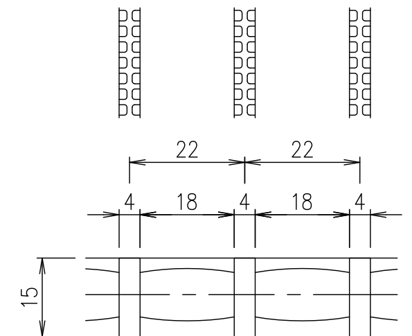
メンバーピッチ詳細図 S=1/1
