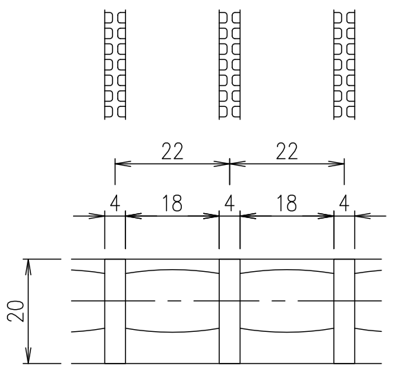
メインバーピッチ詳細図 S=1/1
