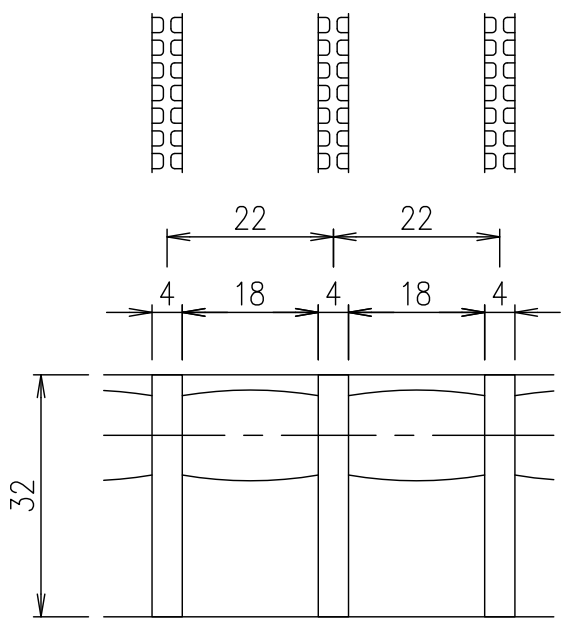
メインバーピッチ詳細図 S=1/1
