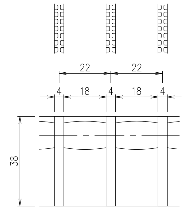
メンバーピッチ詳細図 S=1/1
