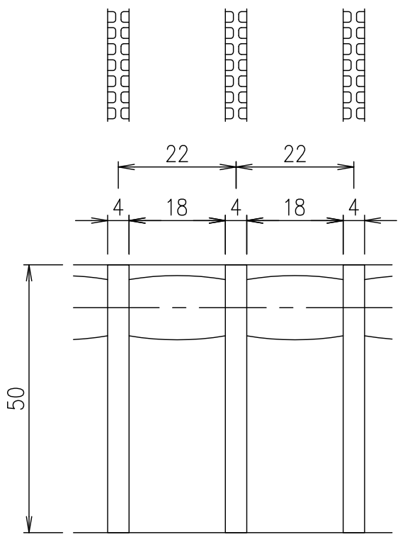
メインバーピッチ詳細図 S=1/1
