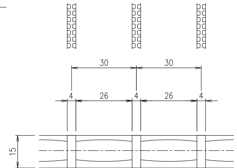
メンバーピッチ詳細図 S=1/1
