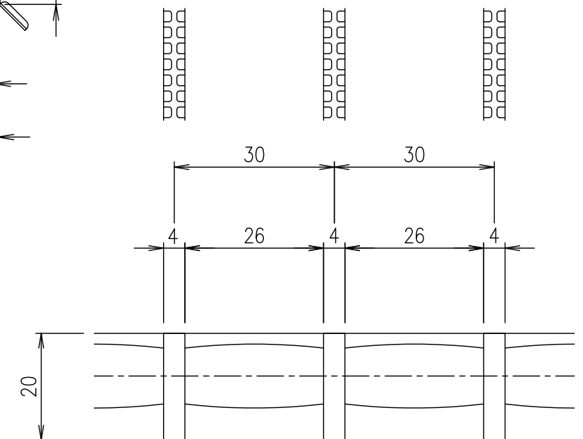
メンバーピッチ詳細図 S=1/1
