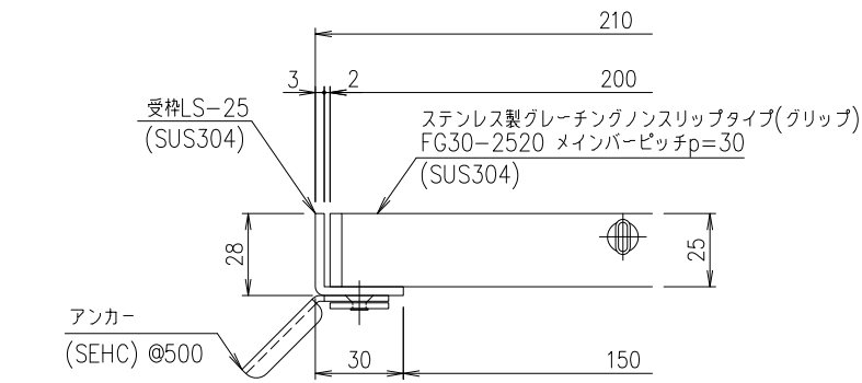
受枠断面詳細図 S=1/2
