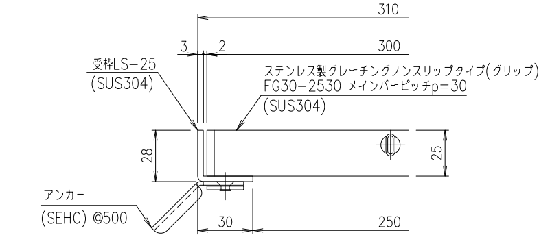
受枠断面詳細図 S=1/2
