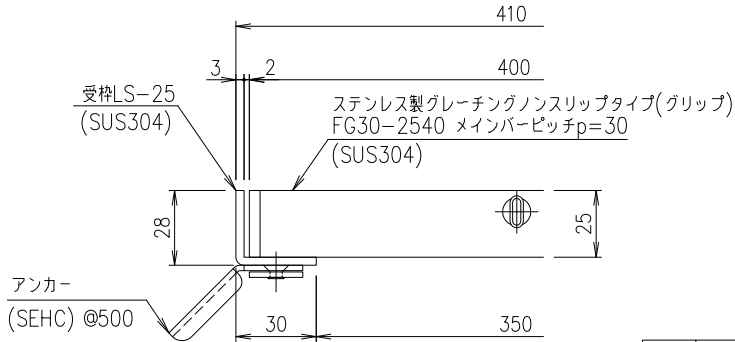
受枠断面詳細図 S=1/2
