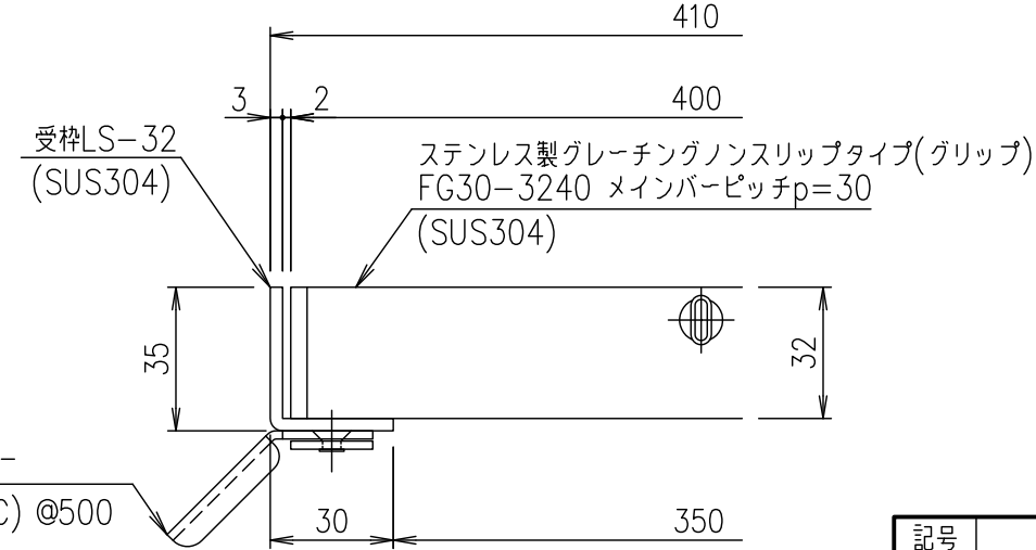
受枠断面詳細図 S=1/2
