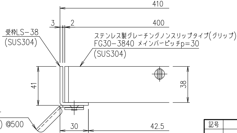
受枠断面詳細図 S=1/2
