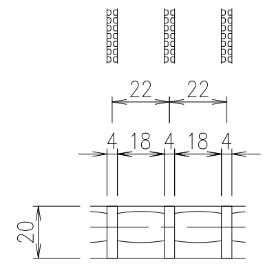
メインバーピッチ詳細図 S=1/2
