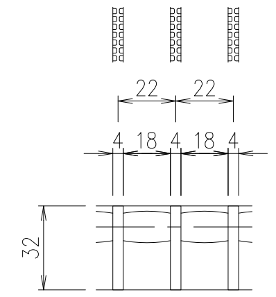
メンバーピッチ詳細図 S=1/2
