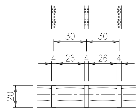
メインバーピッチ詳細図 S=1/2
