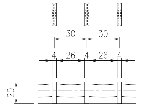
メインバーピッチ詳細図 S=1/2
