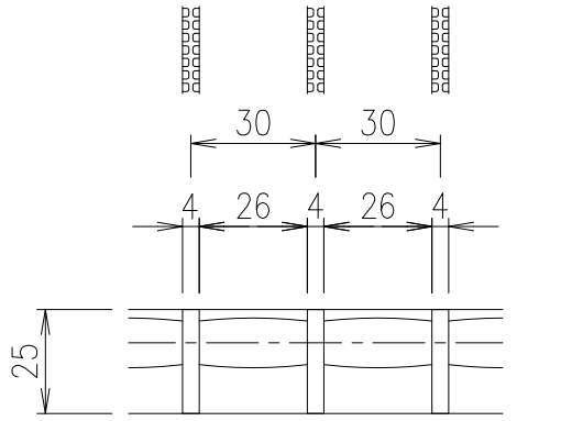
メインバーピッチ詳細図 S=1/2
