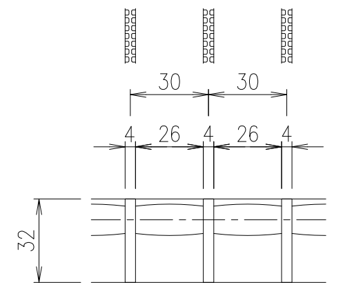
メインバーピッチ詳細図 S=1/2
