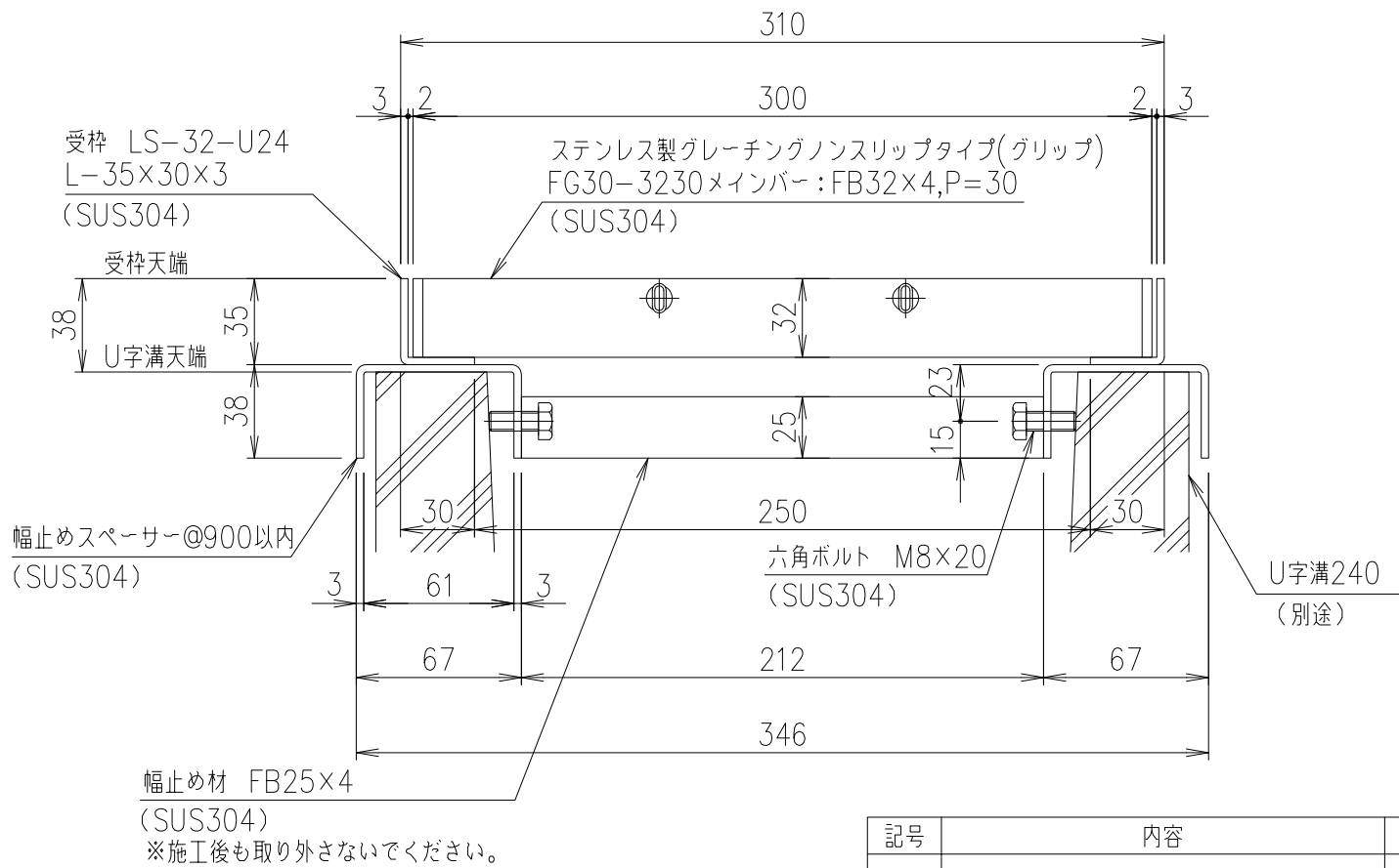
断面詳細図 S=1/3
