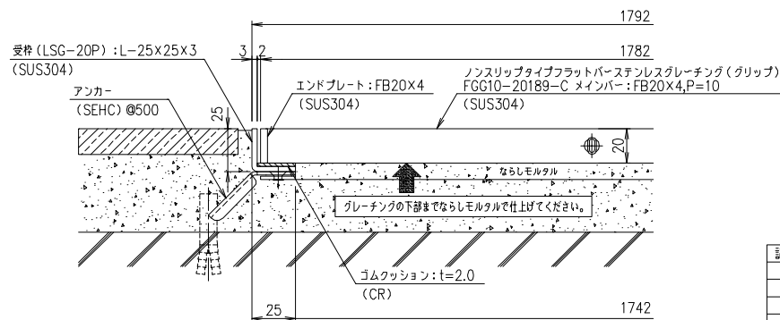
断面詳細図 S=1/2
