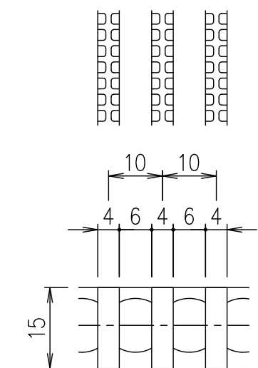
メンバーピッチ詳細図 S=1/1
