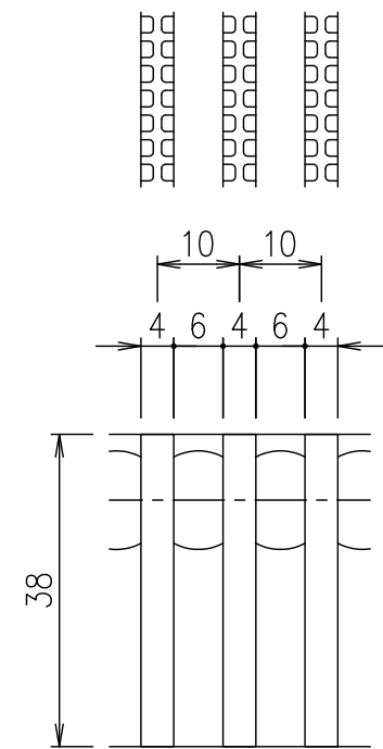
メンバーピッチ詳細図 S=1/1
