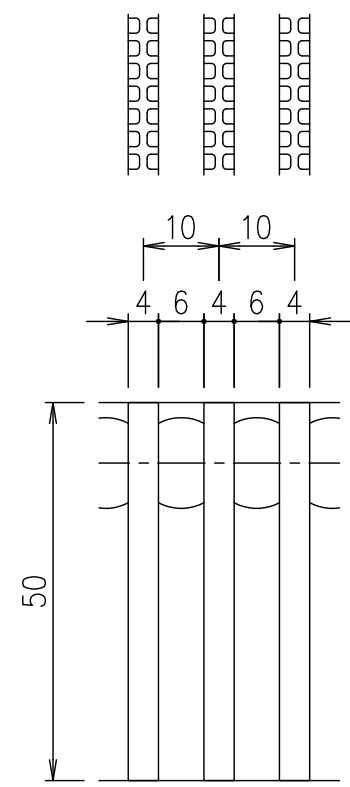
メインバーピッチ詳細図 S=1/1
