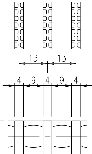
メインバーピッチ詳細図 S=1/1
