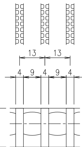
メインバーピッチ詳細図 S=1/1
