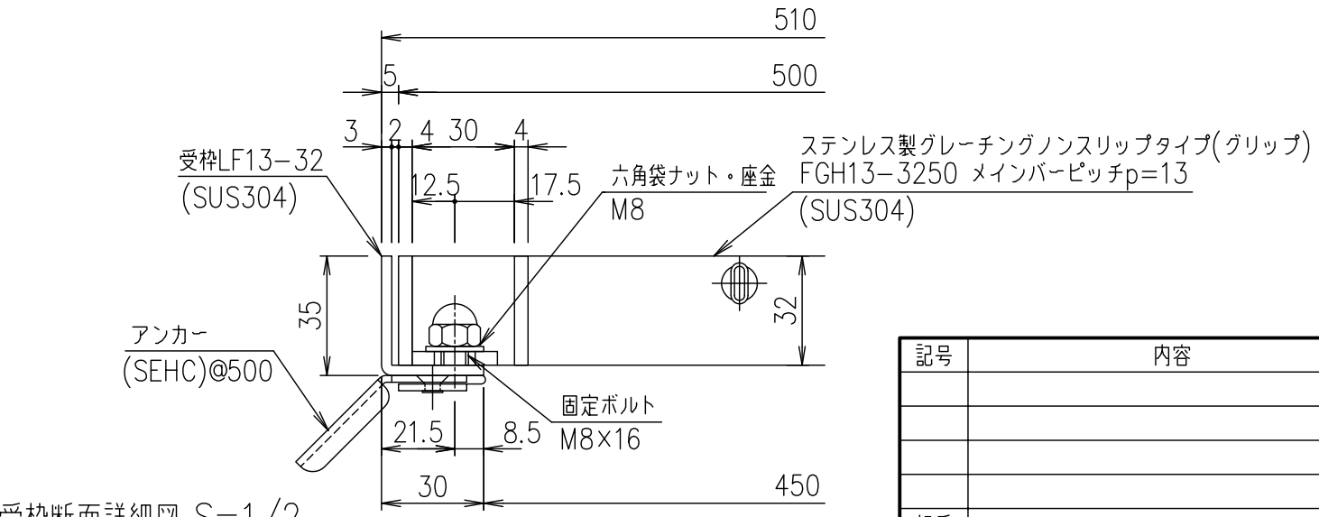
受枠断面詳細図 S=1/2
