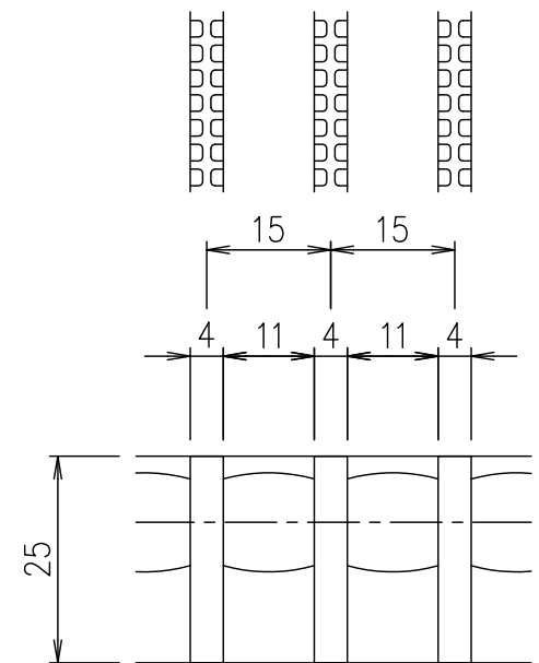
メンバーピッチ詳細図 S=1/1
