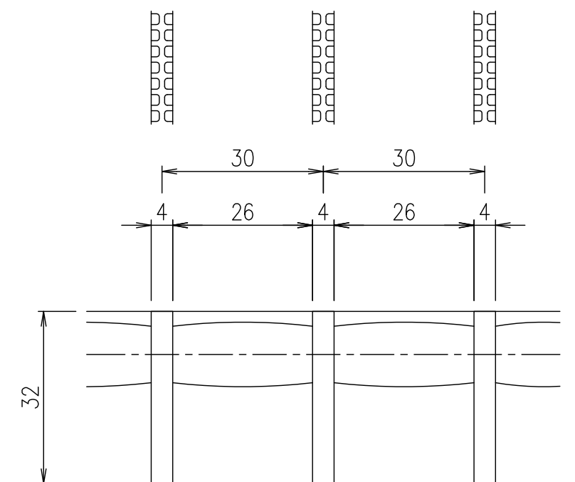
メンバーピッチ詳細図 S=1/1
