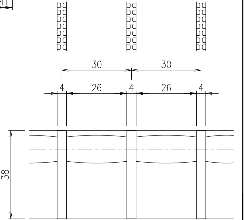
メインバーピッチ詳細図 S=1/1
