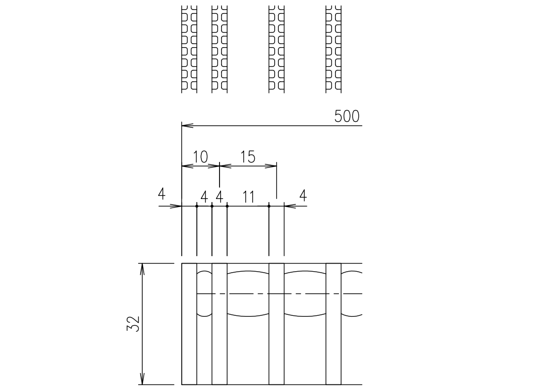
メインバーピッチ詳細図 S=1/1
