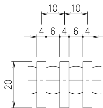
メインバーピッチ詳細図 S=1/1
