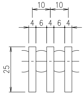
メインバーピッチ詳細図 S=1/1
