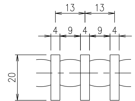
メンバーピッチ詳細図 S=1/1
