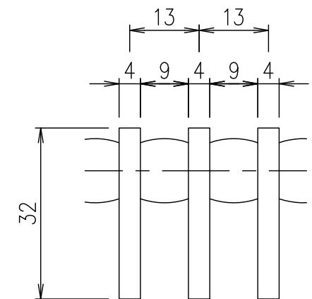
メンバーピッチ詳細図 S=1/1
