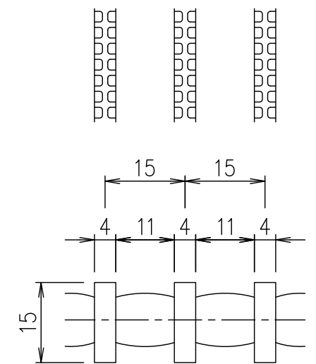
メンバーピッチ詳細図 S=1/1
